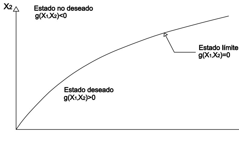
Figura C.1 Representación de la función g(\underline{X}) para el caso con dos variables básicas X_1 y X_2 ; \underline{X} = (X_1, X_2)
