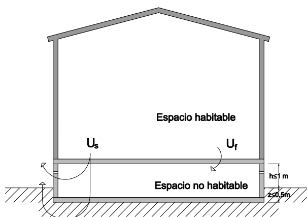
Figura 3.8. Cámaras sanitarias
