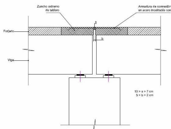
b) articulación entre losas de conexión con pasadores
