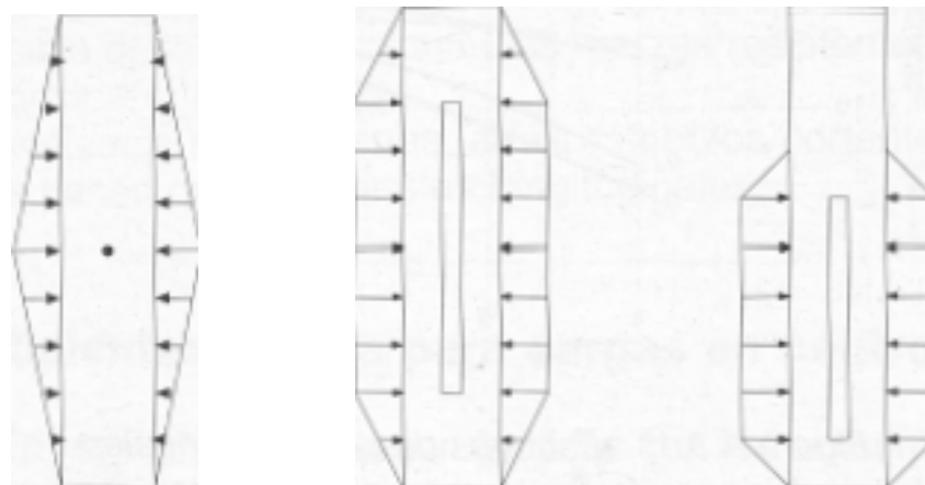
Figura A.12.5.2.4.c. Factores de distribución de carga para cargas puntuales en el borde ( b=1,20 m)
