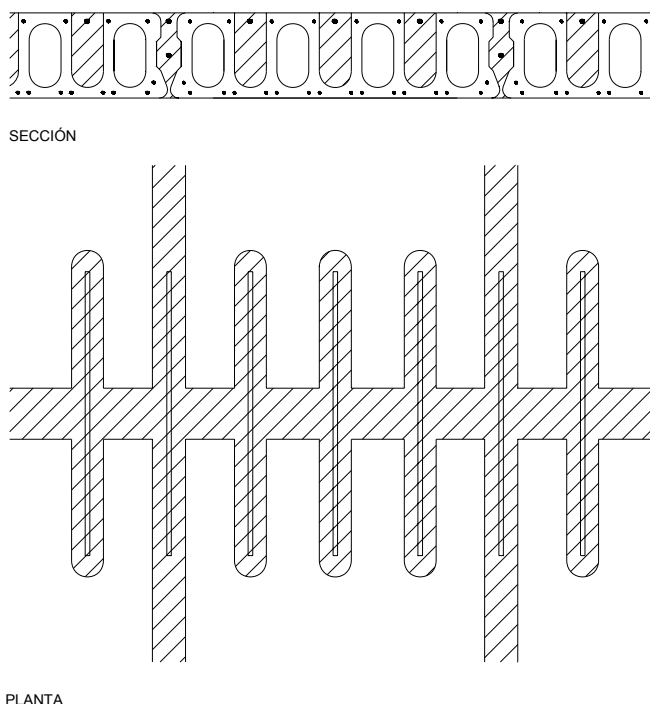
Figura 59.2.4.a Armadura superior en losas alveolares pretensadas
