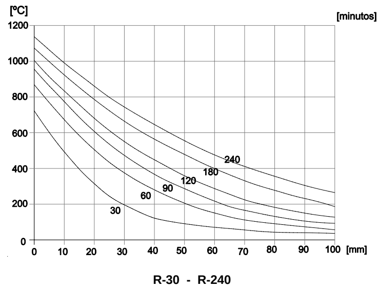
Figura A.6.7.4.c. Distribución de temperaturas en el espesor de secciones planas expuestas por una cara h \geq 200 mm
