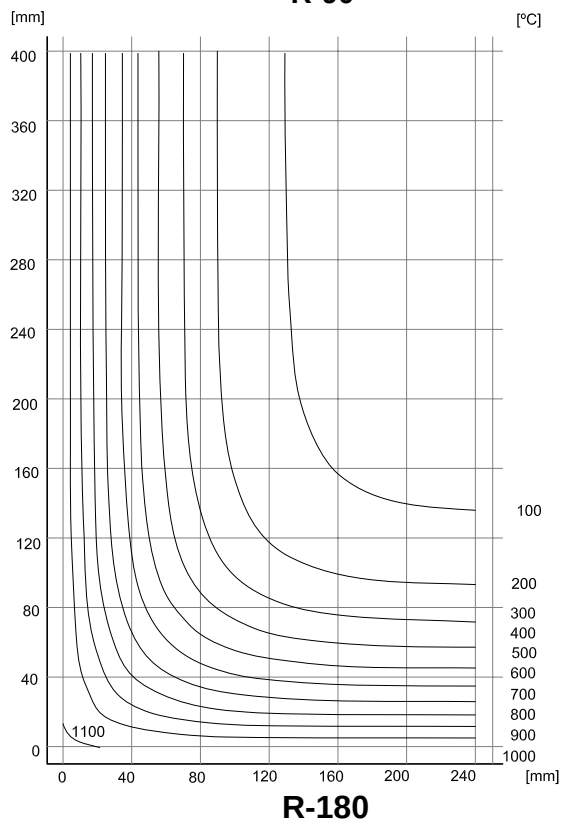
Figura A.6.4.c. Isotermas para cuartos de sección de 800 x 500 mm expuestos por ambas caras
