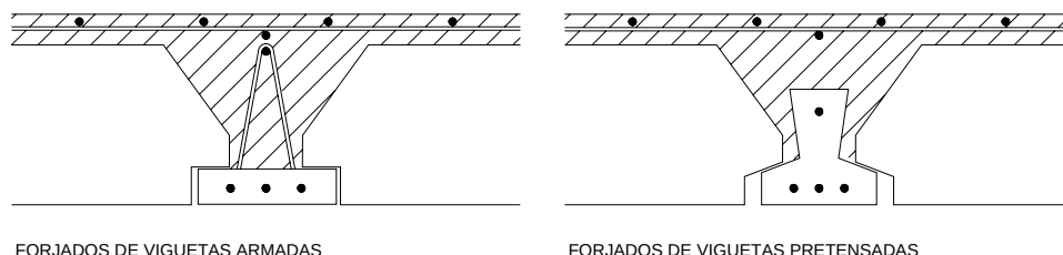
Figura A.12.3.1. Tipos usuales de forjados de viguetas
