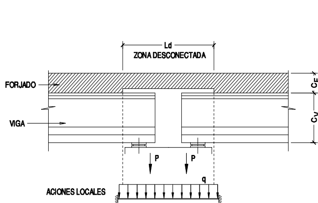
a) Losa de continuidad entre tableros
