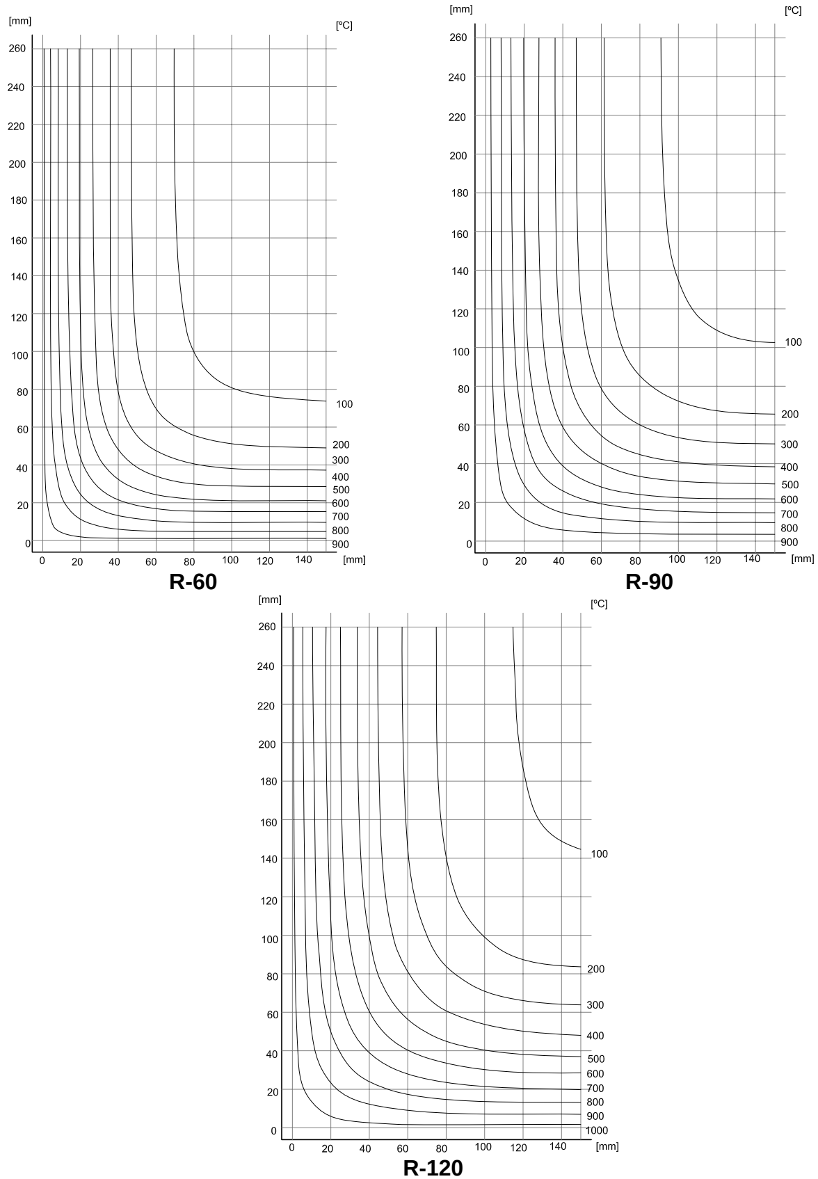
Figura A.6.4.b. Isotermas para cuartos de sección de 600 x 300 mm expuestos por ambas caras
