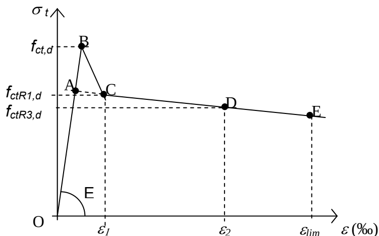
Figura A.14.3. Diagrama de cálculo multilinear.
